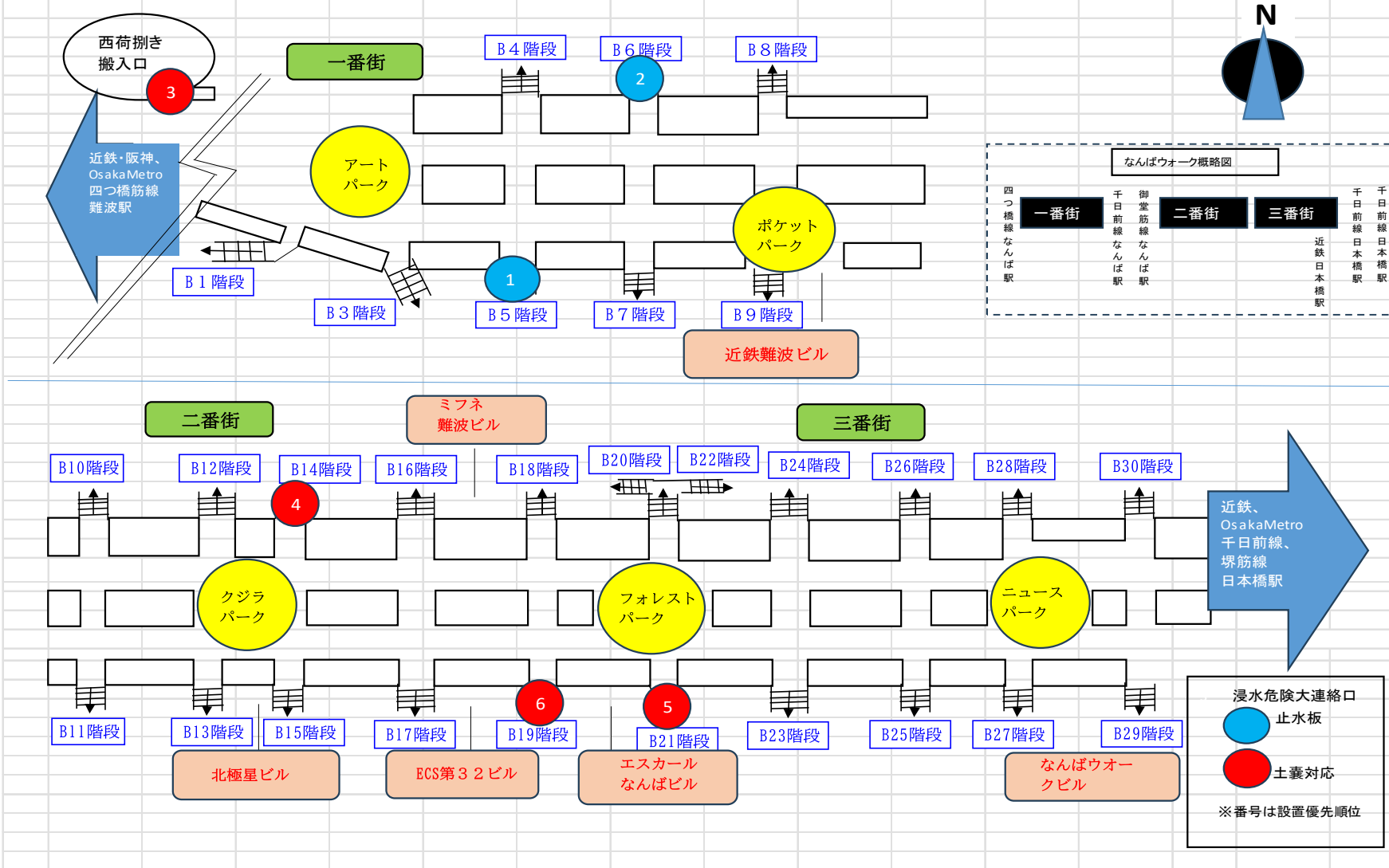
なんばウオーク平面図(地上連絡口、接続・隣接施設接続口)
